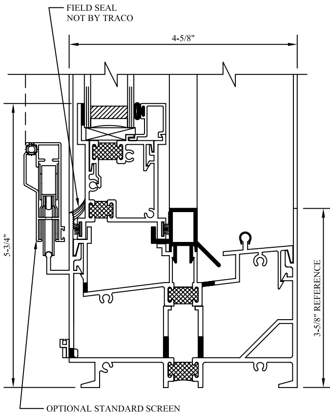
OPTIONAL 12 PSF SILL
