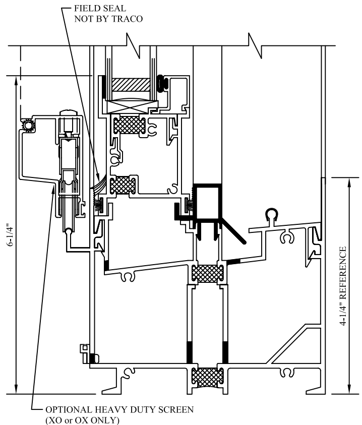
OPTIONAL 15 PSF SILL
