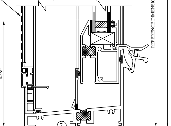
7 SILL (BEVEL SASH)
