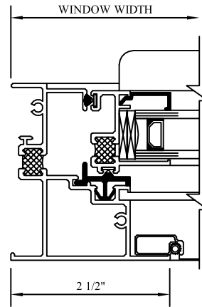
④ JAMB
